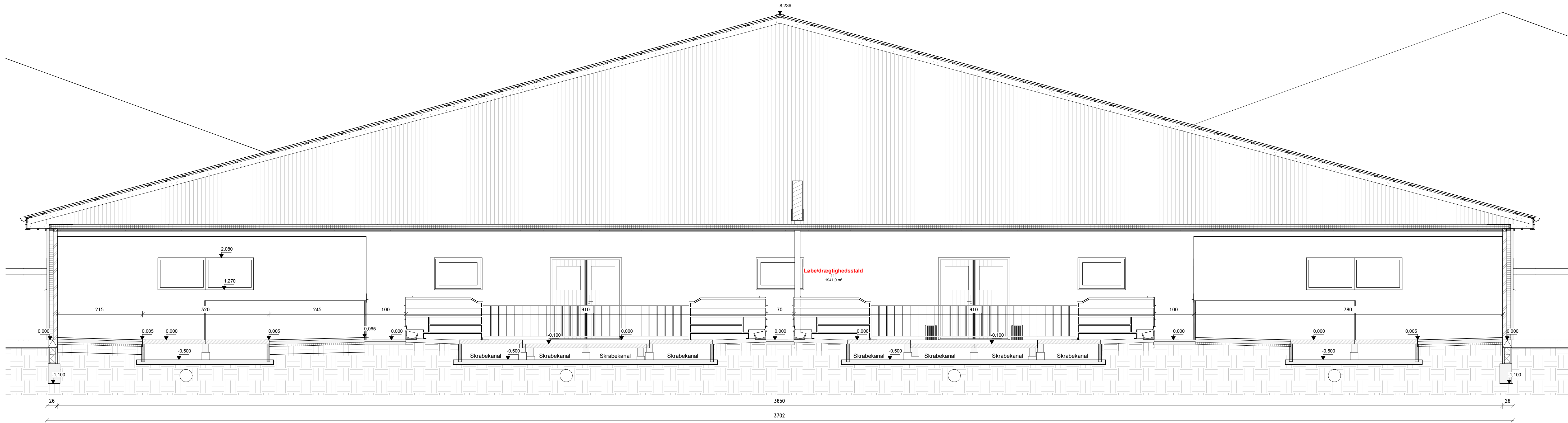
Principsnit A4, 1 : 50
