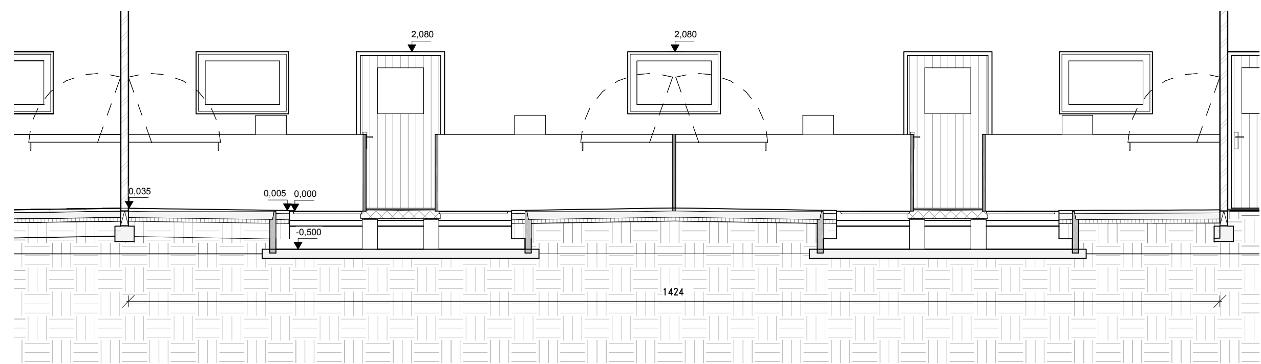
Principsnit B, 1 : 50
