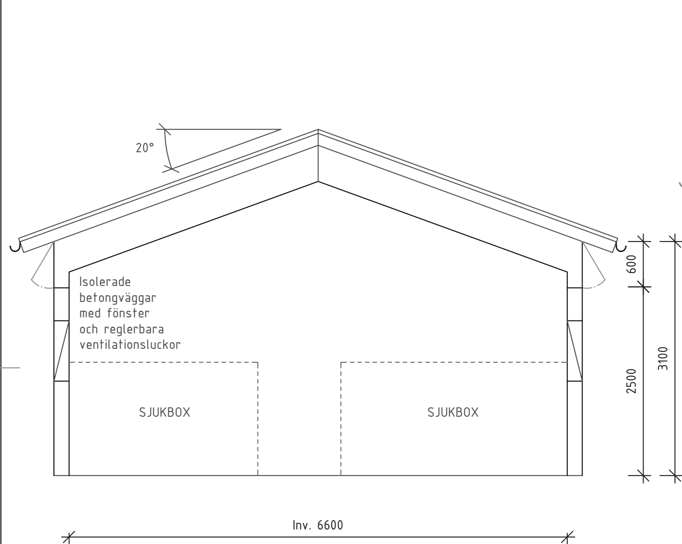
SEKTION E-E
