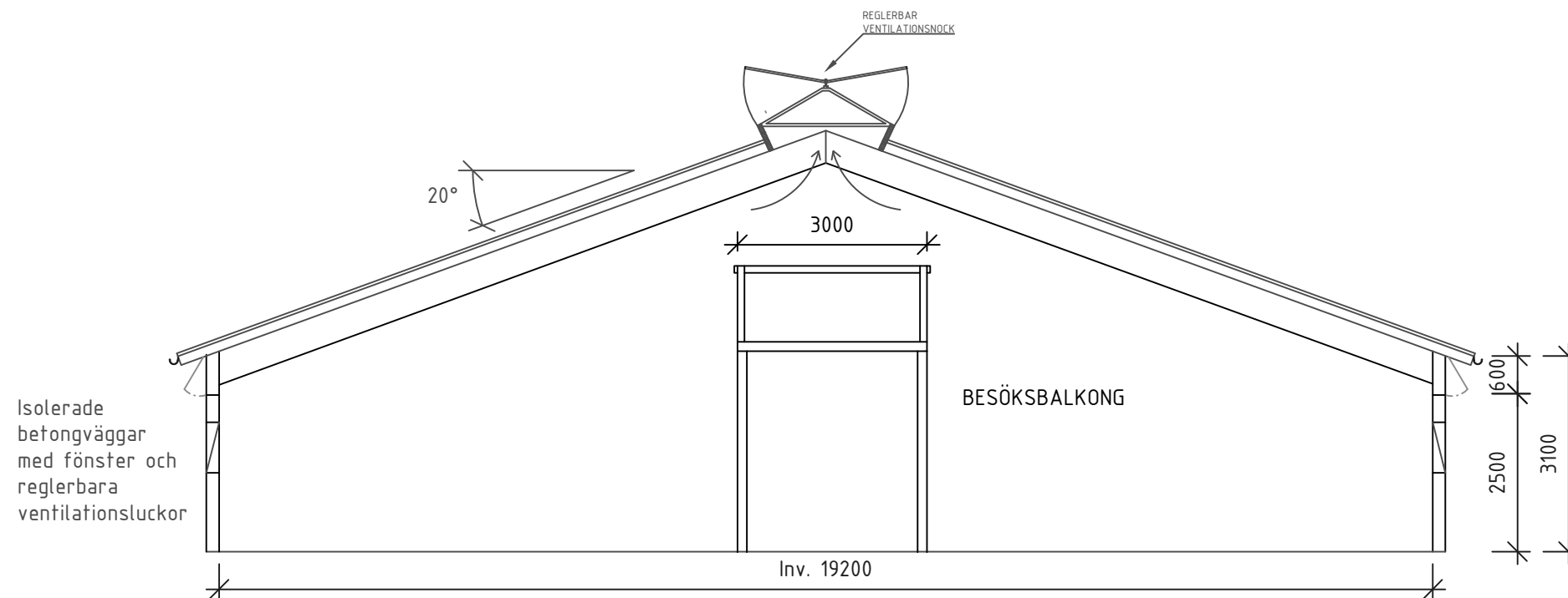
SEKTION D-D
