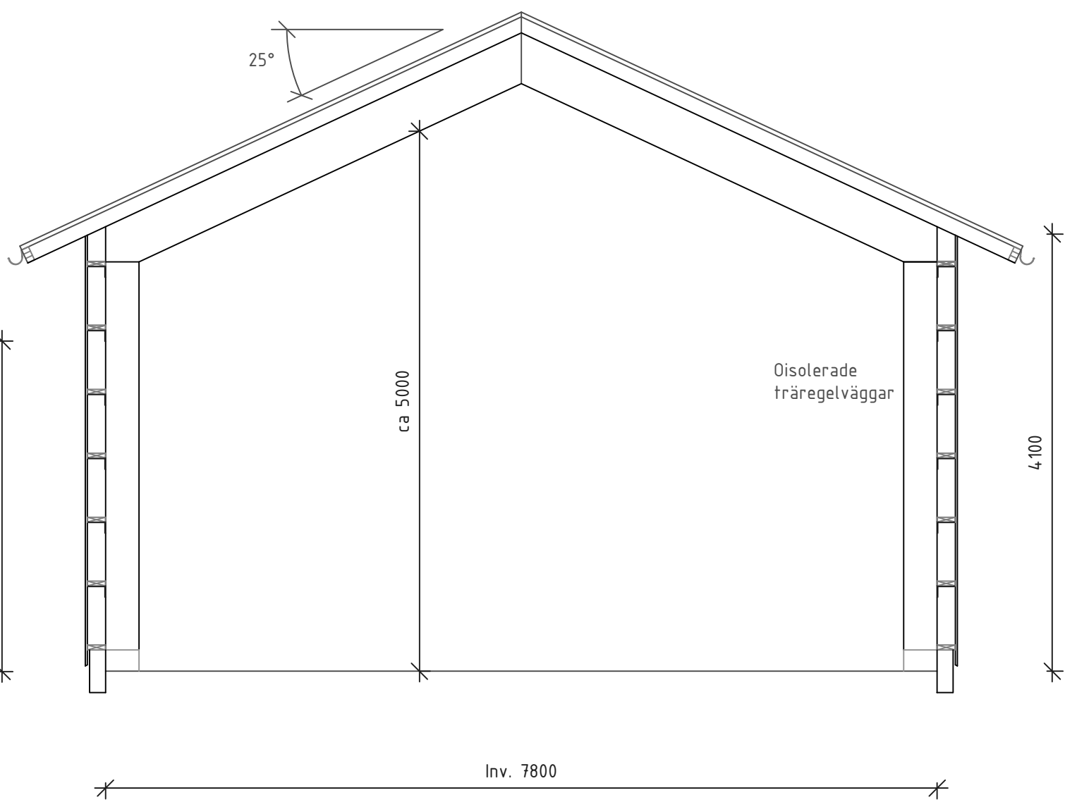
SEKTION F-F
