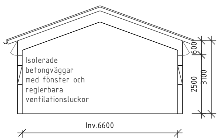
SEKTION E-E
