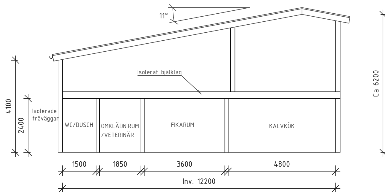
SEKTION B-B
