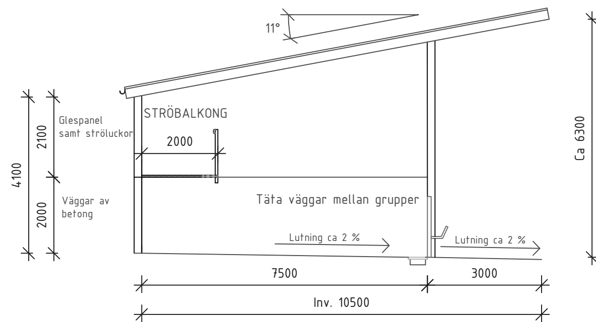
SEKTION A-A
